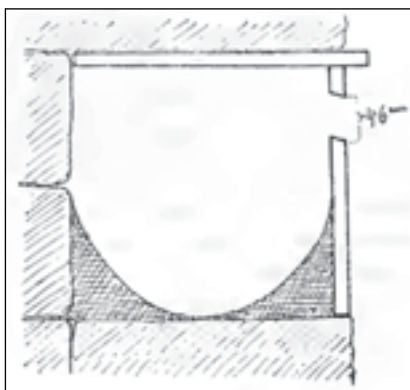
Téglarésodú (Aquila, 16. évf. 1-4. sz. 1909. 213.)
