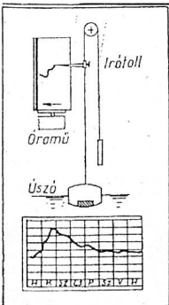
A rajzoló vízmérce elvi vázlatja és a grafikon
